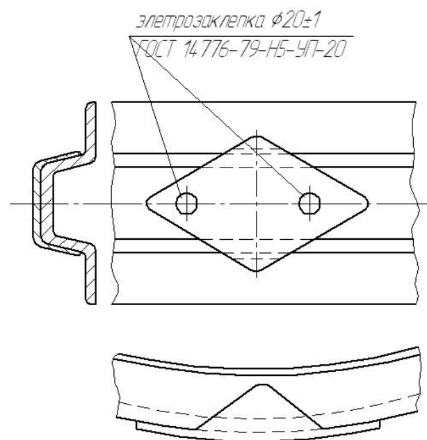
Рисунок 16. Примерное расположение усиливающей накладки на шпангоуте (при наличии трещины на горизонтальной полке, переходящей на вертикальные стенки)
