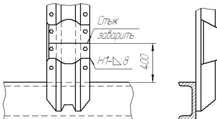
Рисунок 18 Ремонт стоек с изломом
