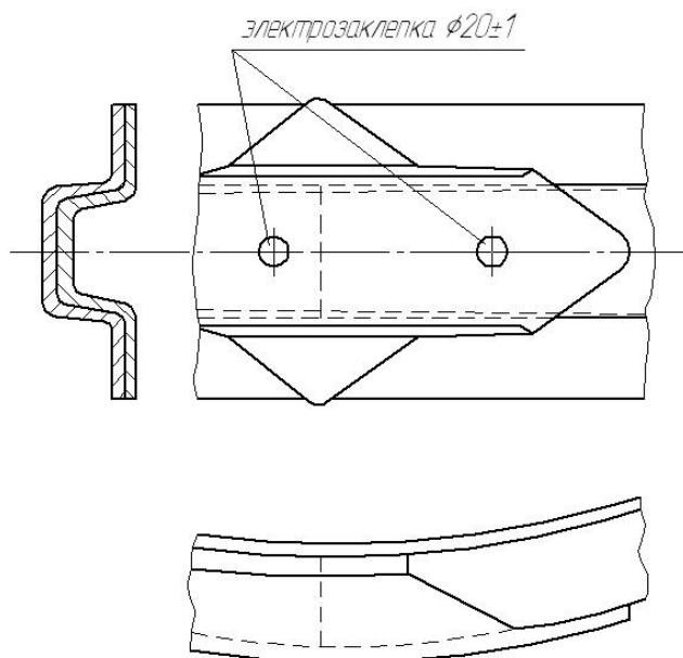
Рисунок 17. Расположение усиливающей накладки на фланце (при наличии трещины на горизонтальной полке)
