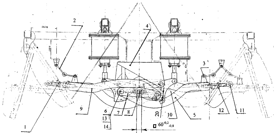
Рисунок 22. Привод механизма разгрузки
