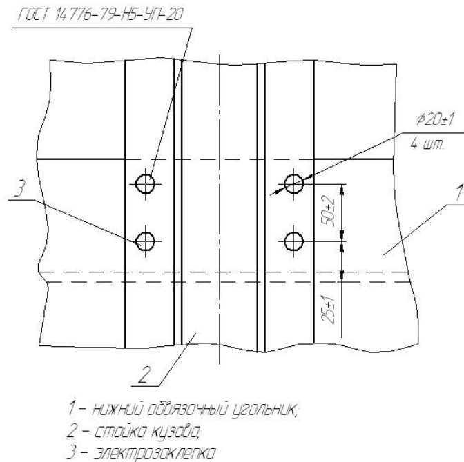
Рисунок 6. Дополнительное крепление стойки электрозаклепками
