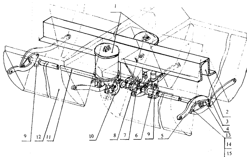
Рисунок 22. Привод механизма разгрузки
