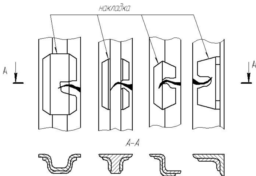
Рисунок 7. Варианты ремонта стоек кузова
