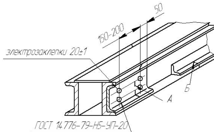
Рисунок 2 Ремонт хребтовой балки цистерны
