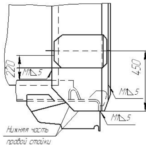
Рисунок 2 Ремонт хребтовой балки цистерны
