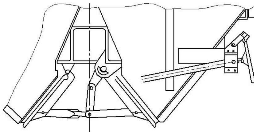
Рисунок 29. Механизм разгрузки вагона для зерна постройки 1976-1979г.
