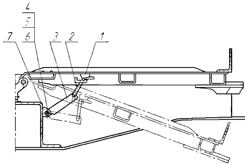
1 - опора, 2 - торсион, 3 - рычаг, 4 - валик, 5 - шайба, 6 - шплинт, 7 - ушко
