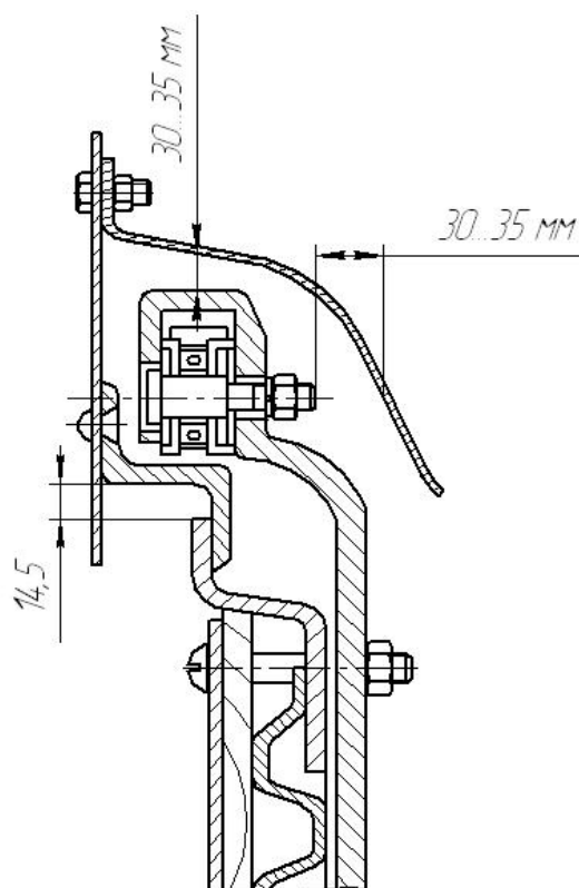
Рисунок 21. Размер перекрытия зонтом верхней части двери
