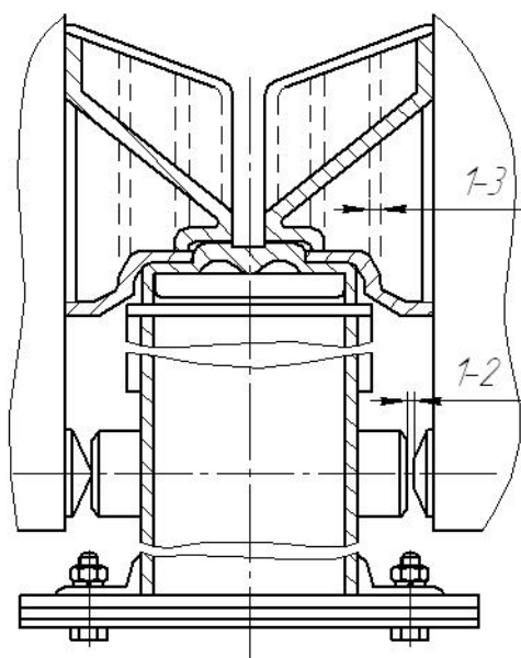
Рисунок 32 Установка бункеров модель 17-409 и 17-431.
