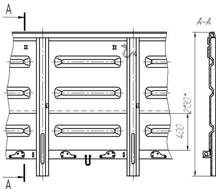
Рисунок 8. Схема замены части обшивки
