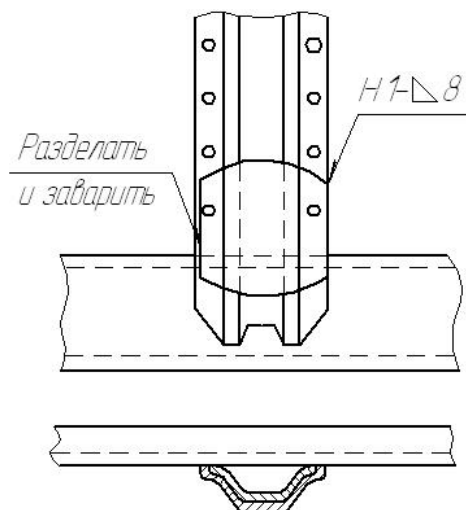
Рисунок 18а. Заварка трещин на стойках кузова
