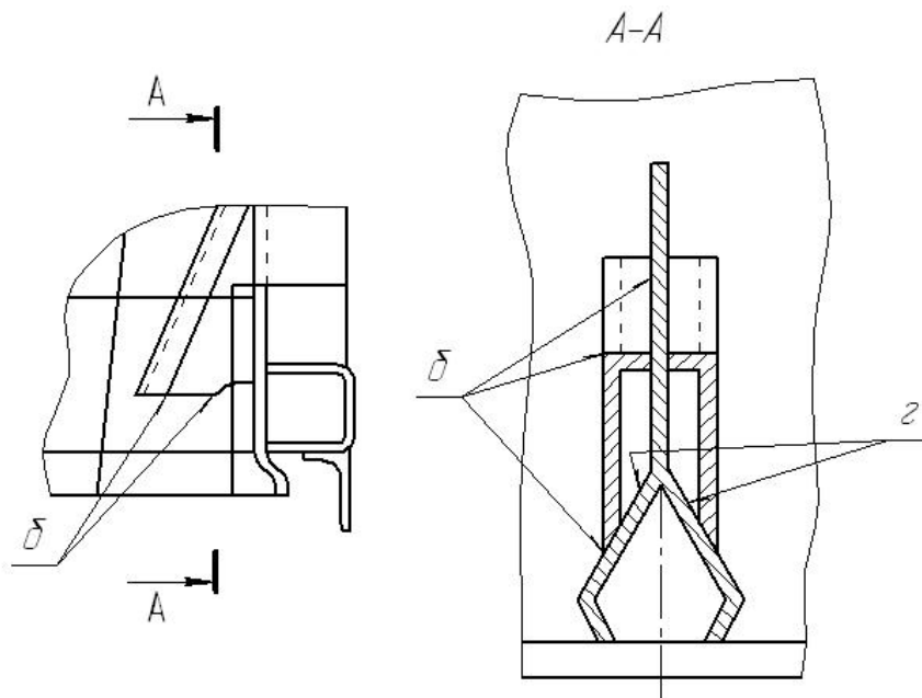
Рисунок 26. Усиливающие накладки на промежуточных балках.
