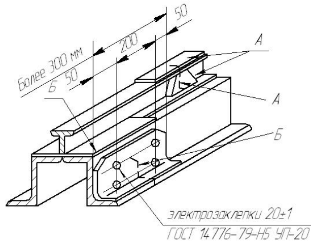
Рисунок 1 Ремонт хребтовой балки полувагона
