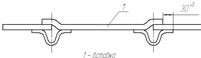
Рисунок 4. Установка вставки металлической обшивки
