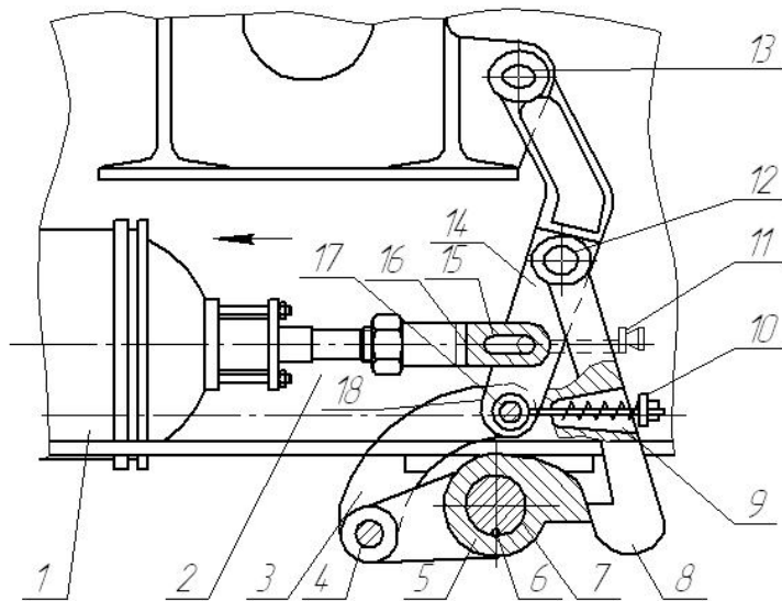
1 - цилиндр, 2 - шток, 3, 14 - рычаги, 4, 12, 13, 15, 17 - валики, 5 - рычаг поворота, 6 - шпонка, 7 - вал, 8 - защелка, 9 - пружина, 10 - тяга, 11 - винт, 16 - головка штока, 18 - втулка
