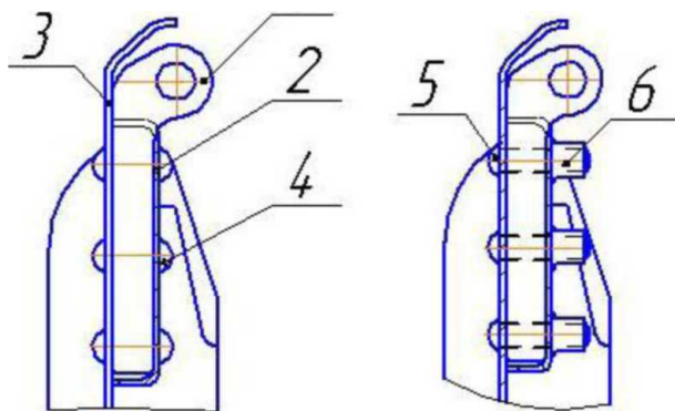
1 - Петля, 2 - Усиление заднее, 3 - Лист крышки люка, 4 - Заклепка, 5 - Штифт с полукруглой головкой, 6 - Головка обжимная
