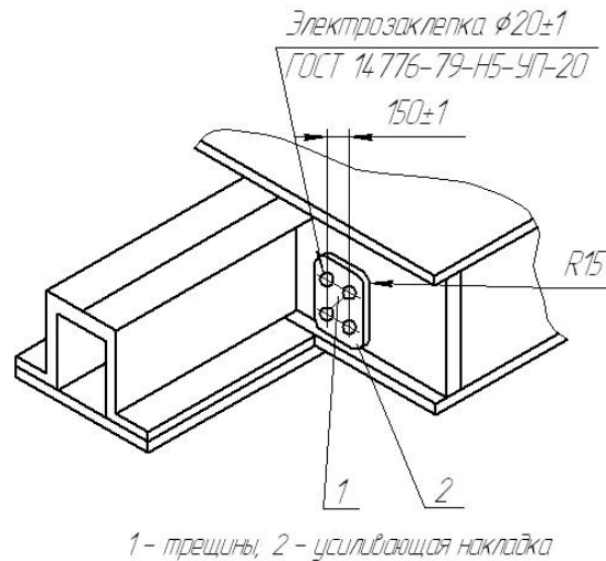
Рисунок 15 Ремонт диафрагм шкворневых балок с помощью усиливающих накладок
