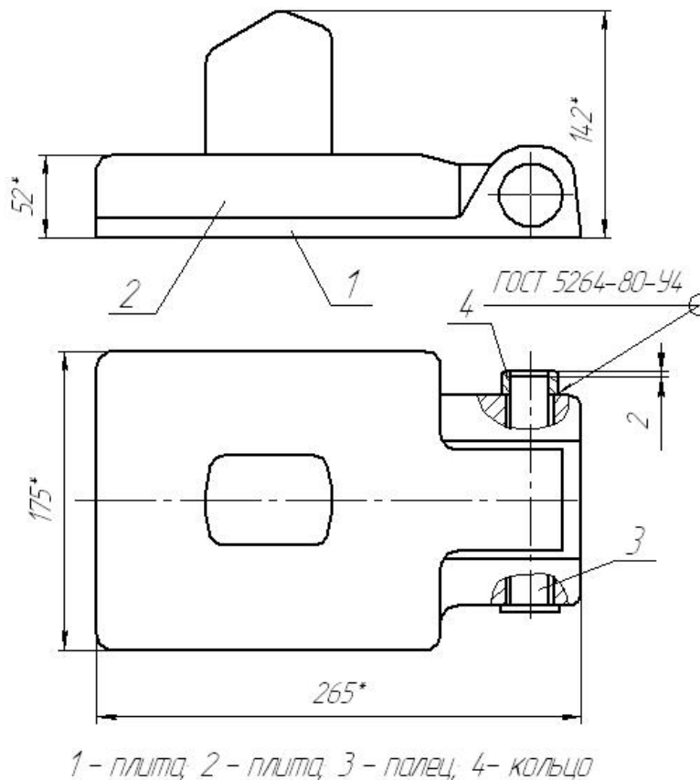
Рисунок 35. Плита с упором
