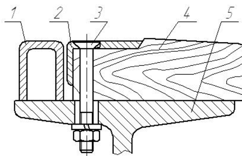
1-предохранитель брус, 2-армированный уголок, 3 болт с потайной головкой, 4-доска пола, 5-продольная балка рамы.
