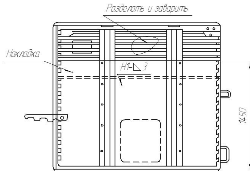
Рисунок 20. Ремонт дверей
