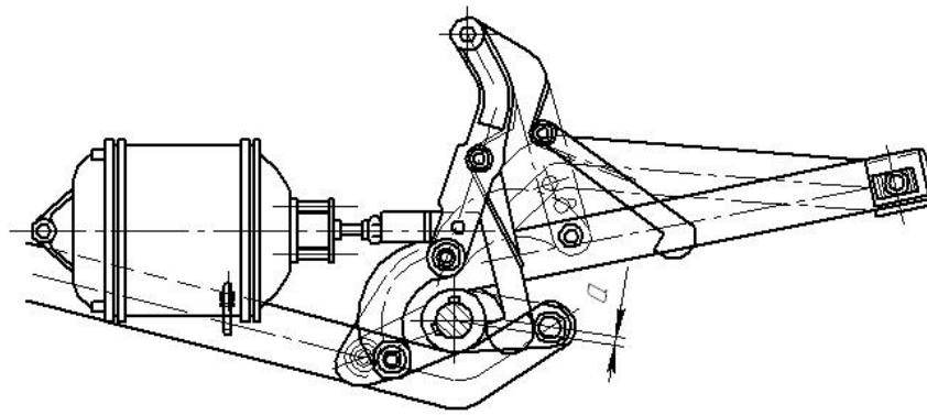
Рисунок 13. Механизм разгрузки
