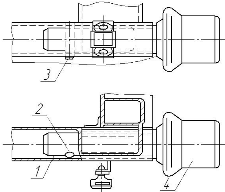
1-ось бегунка, 2-стопорная ось, 3-шплинт, 4-бегунок
