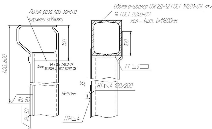
Рисунок 4. Установка вставки металлической обшивки
