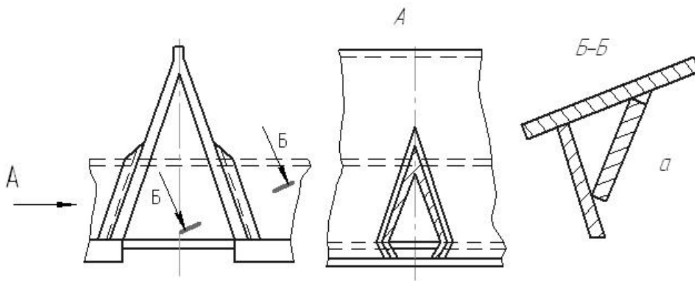
Рисунок 25. Усиливающие накладки на продольной балке.
