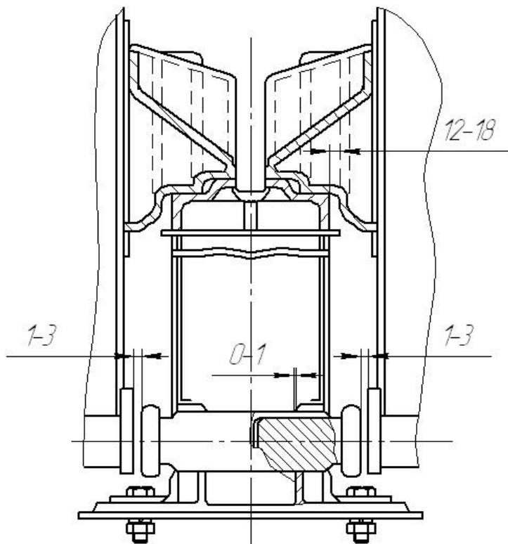
Рисунок 31 Установка бункеров модель 17-494.
