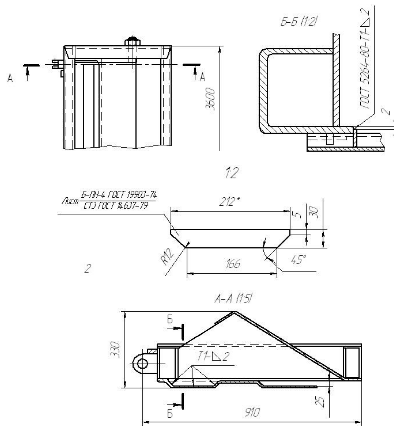
Рисунок 12 Заварка отверстия в крышке люка полувагона-хоппера для перевозки горячих окатышей
