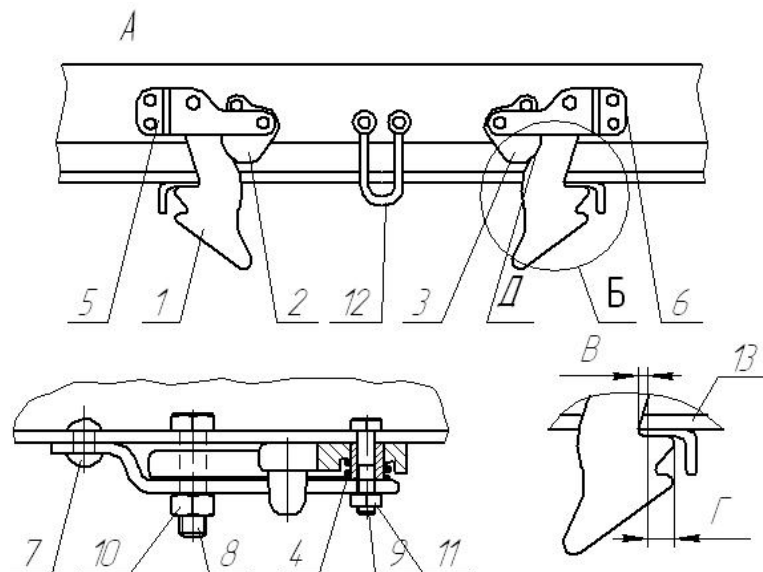
1-закидка, 2-сектор левый, 3-сектор правый, 4-пружина, 5-скоба левая, 6-скоба правая, 7-заклепка, 8,9 -болт, 10,11-гайка, 12-скоба, 13-кронштейн крышки люка
