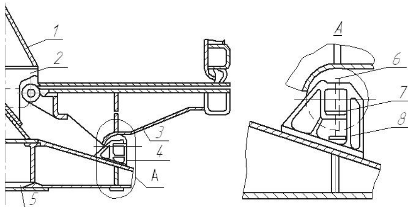
1 - балка кузова, 2 - опора кузова, 3 - крышка люка, 4 - кронштейн с роликом, 5 - рама, 6 - регулировочный болт.
