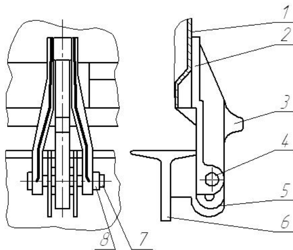
1-дверт, 2-петля, 3-клин, 4-валик, 5-державка, 6-балка, 7-шайба, 8-шплинт
