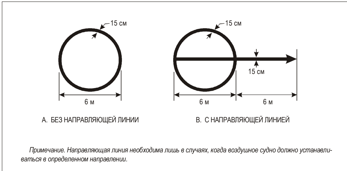
Рис. 5-9. Маркировка аэродромного пункта проверки VOR
